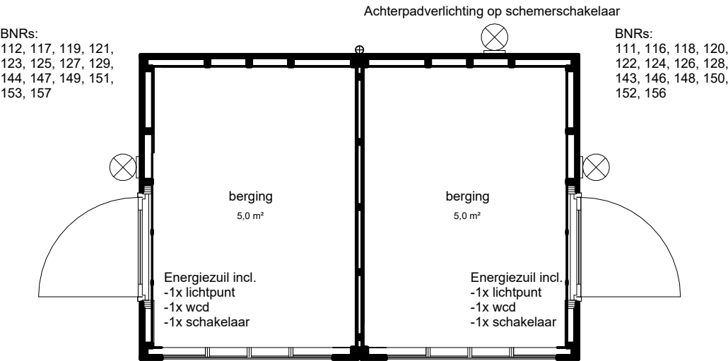
Begane grond
