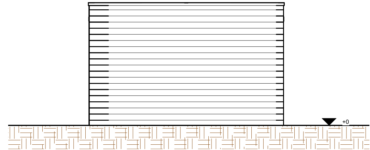
Tuinzijde
